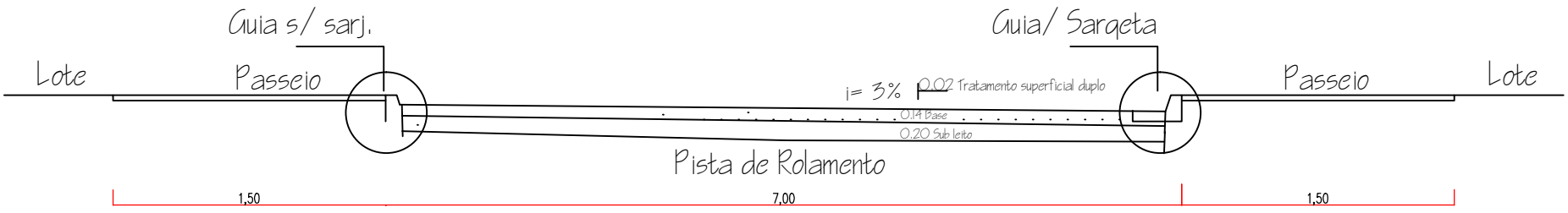
Seções Transversais das Ruas- Rua 01, Rua 02 e Rua 03.
