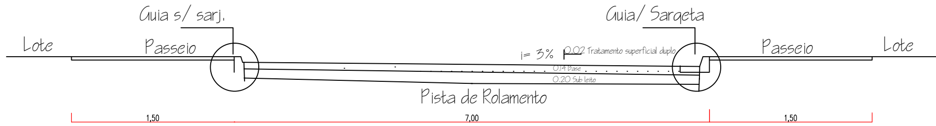
Seções Transversais das Ruas- Rua Francisco Bento Ferreira
