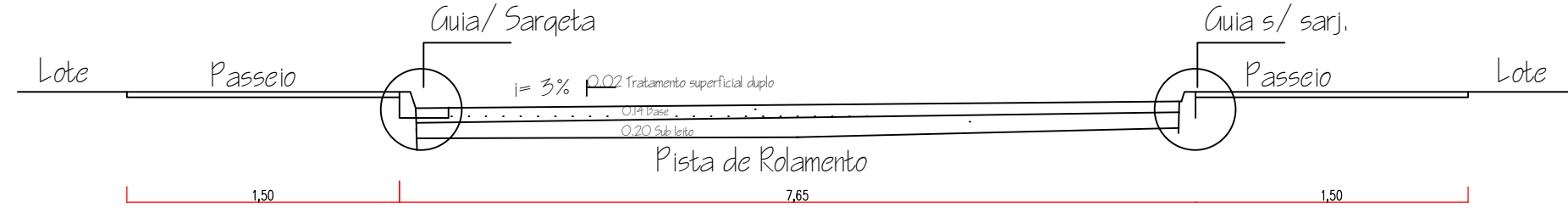
Seções Transversais das Ruas- Rua 04.
